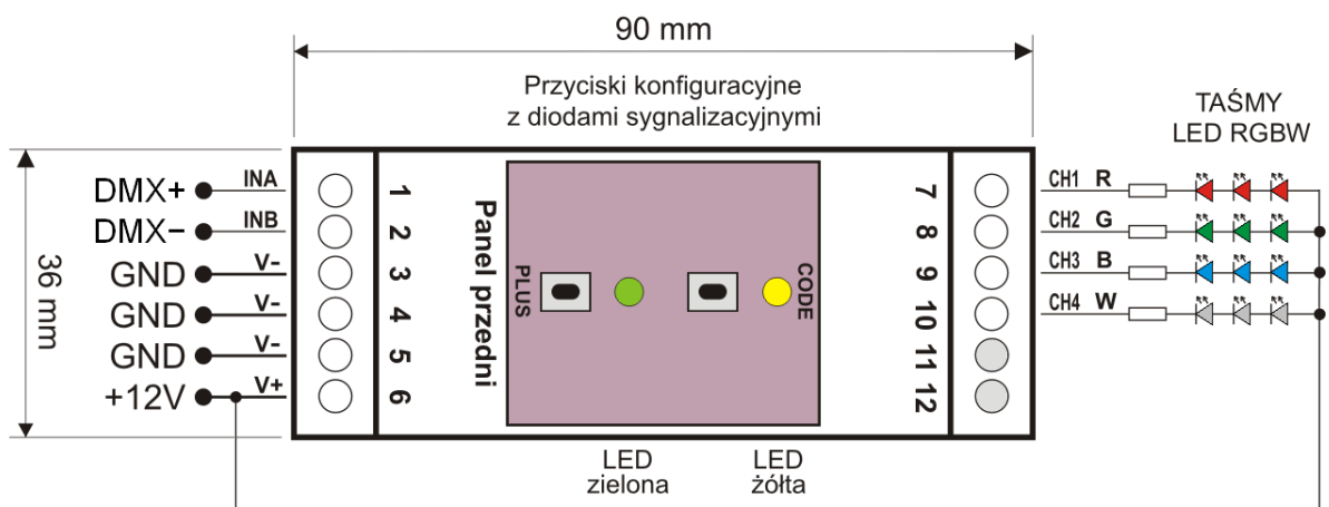
Rys.1. Schemat ogólny i wymiary sterownika SPL-4C.
